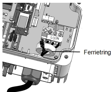
Afbeelding 8: AC-aansluiting
