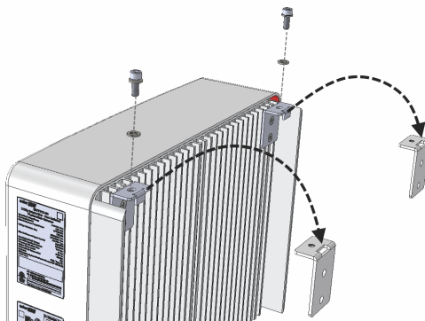
Afbeelding 24: Montagebeugels
