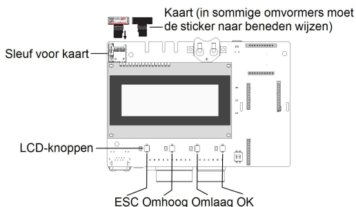
Afbeelding 10: Communicatie-interface en SD-kaart
