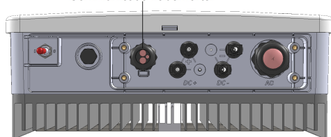
Afbeelding 12: Communicatie-kabelwartel
